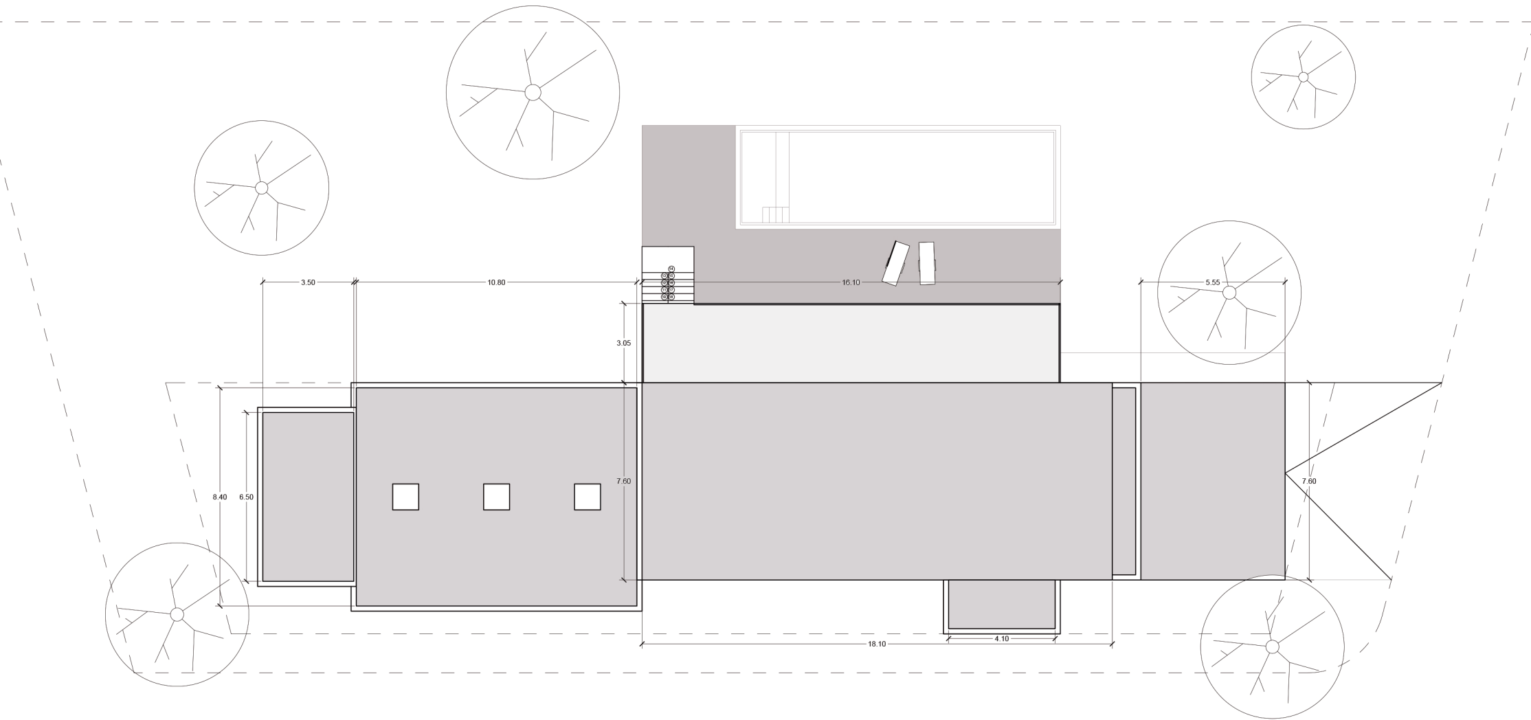
Planta de Cubierta
