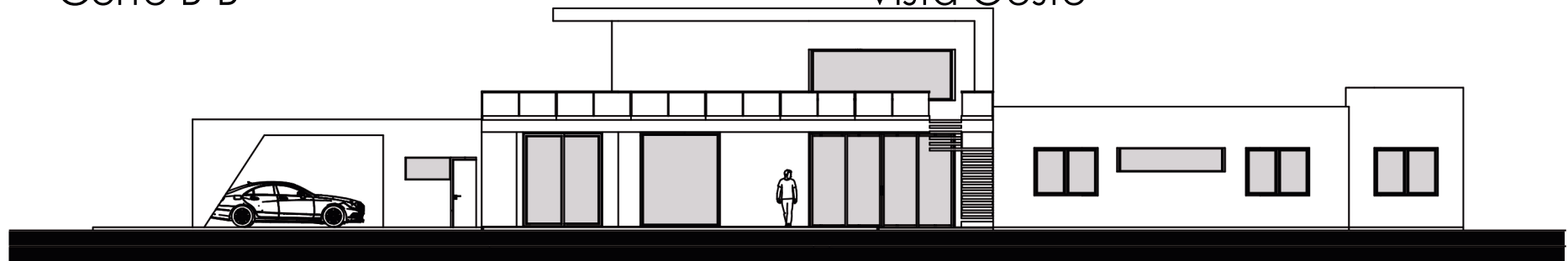
Vista Norte
